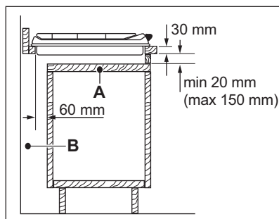
A. Panneau amovible B. Espace pour les branchements
